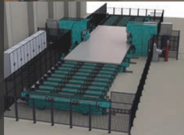
Гибка кромки
