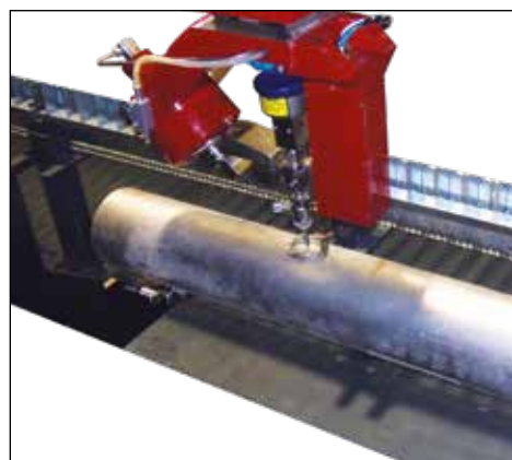
Система резки труб Tube cutting lathe system
